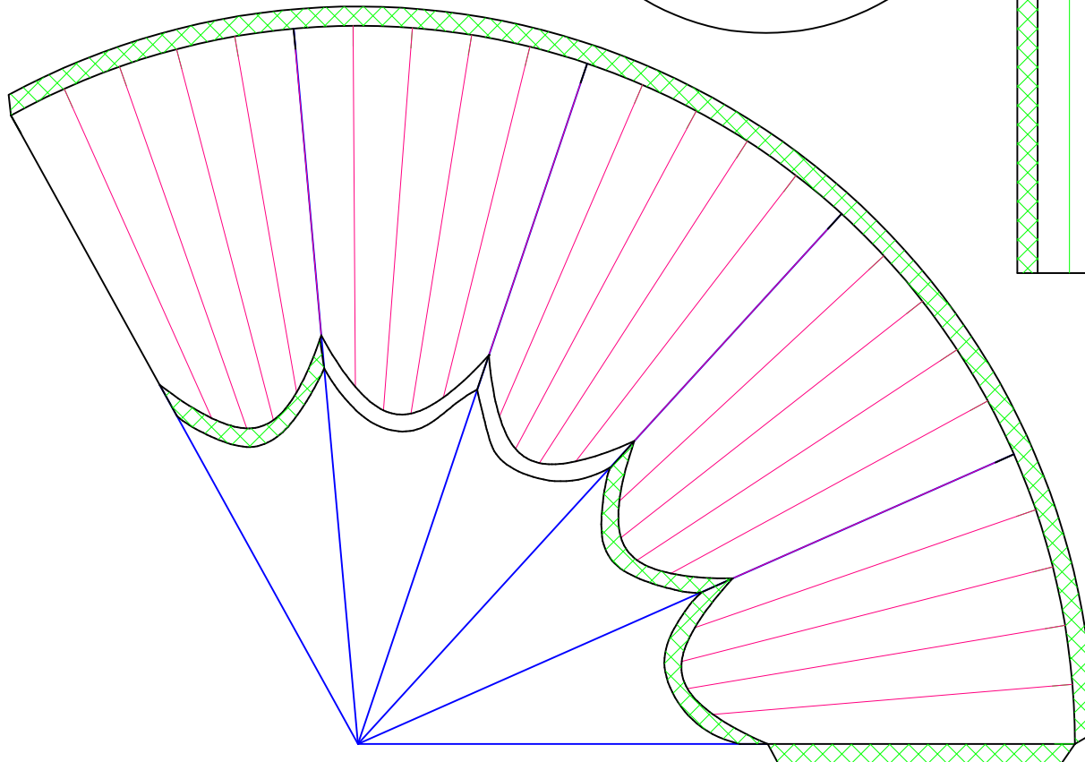
Außenmantel
